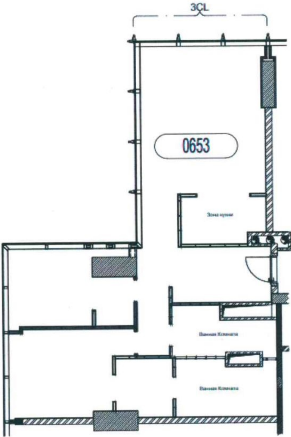
ПЛАН ОБЪЕКТА
